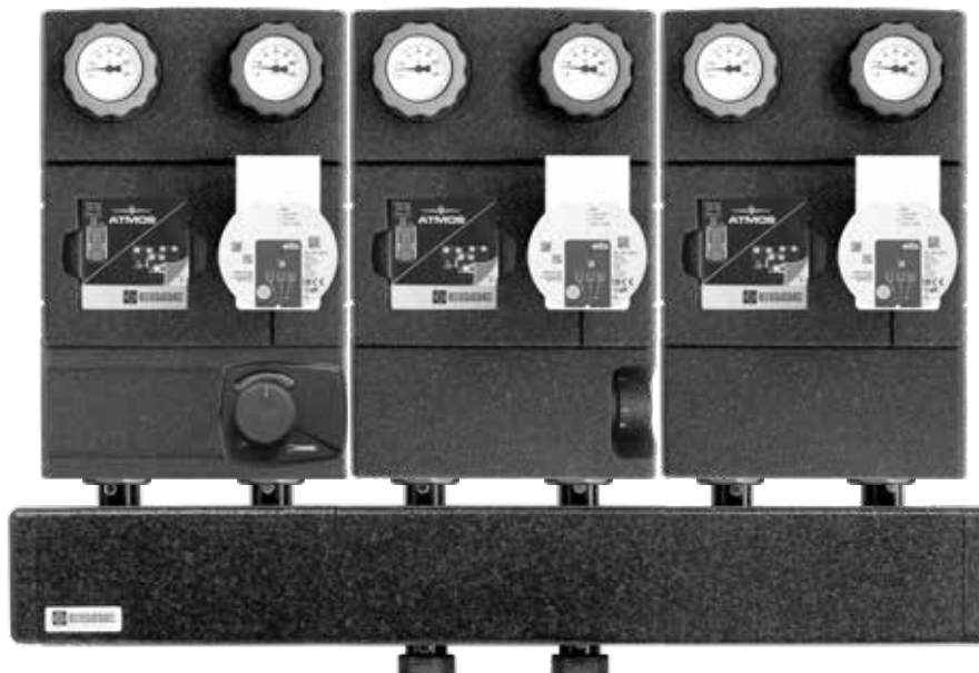
Colector pentru trei unități de circulație (trei circuite)
