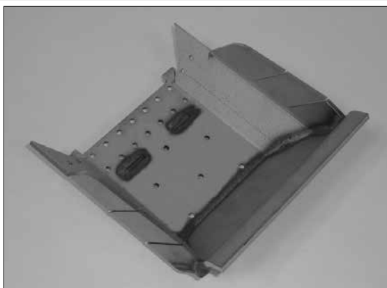
Camera de ardere a arzătorului - pentru curățarea pneumatică
